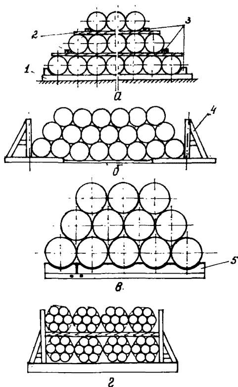
Рис. 9. Способы складирования труб: а - посклойно; б и в - в "седло" (на плоских и желобчатых подкладках); г - пакетами посклойно; 1 - подкладка; 2 - прокладка; 3 - упор; 4 - упор-сграждение; 5 - сборно-разборный стелаж
