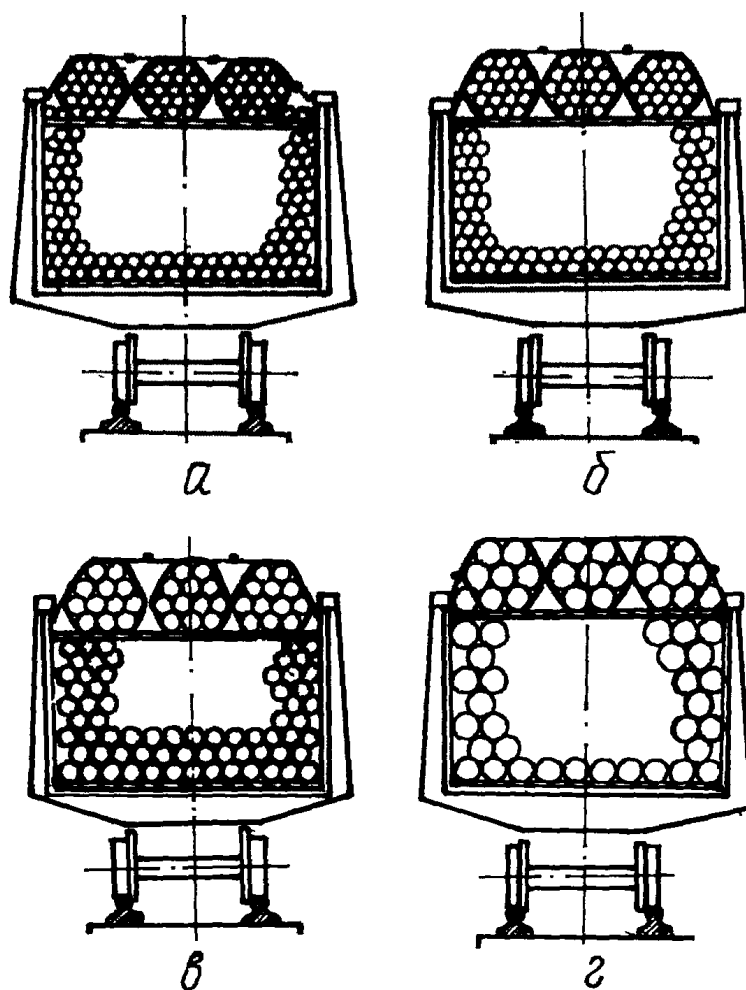
Рис. 4. Схемы комбинированной укладки труб в полувагоны диаметрами:
