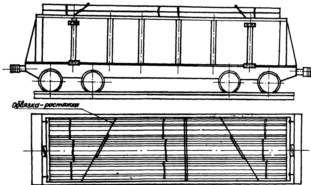
Рис. 6. Схема поперечной обвязки труб в полувагоне
