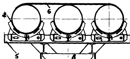
Рис. II. Приспособления для перевозки изолированных труб: а - ПИТ-200; б - ПИ-6 (на автомобиле); в - ПИ-6 (на прицепе-ропускке): 1 - труба; 2 - подкладка; 3 - болт; 4 - брус; 5 - коник; 6 - утяжочный канат
