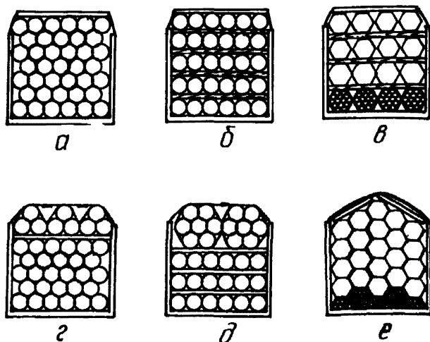
Рис. 1. Схемы размещения труб в полушестигрниках:
