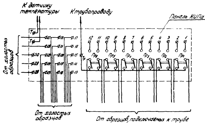
Рис.4. Схема коммутации и электрических соединений на клеммной панели КИП : \phi 1-\phi 32 - номера контактов на схеме; Т-индикация контактов; \Pi p_1-\Pi p_{12} - переключатели
