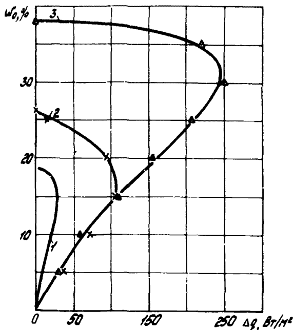
Рис.3. Зависимость эмпирической величины \Delta q от первоначальной влажности грунта w_0 : 1 - n = 0,4 ; 2 - n = 0,47 ; 3 - n = 0,55
