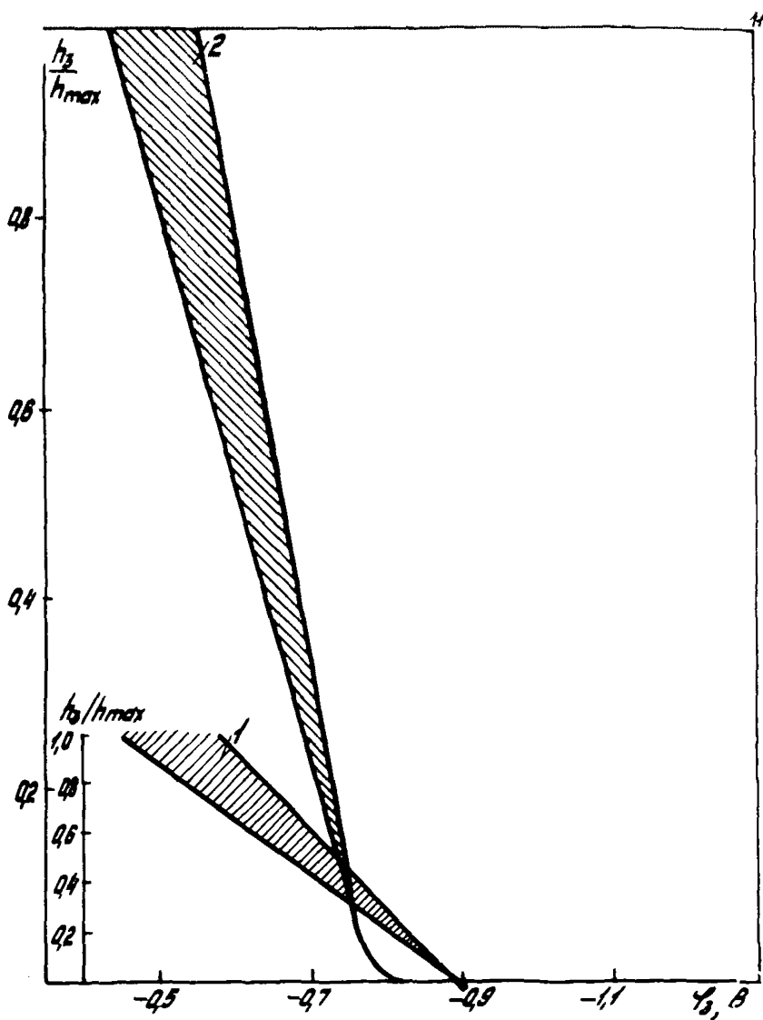
Рис.1. Зависимость величины отношения \frac{h_3}{h_{max}} от величины защитного потенциала для температур стальной поверхности:
