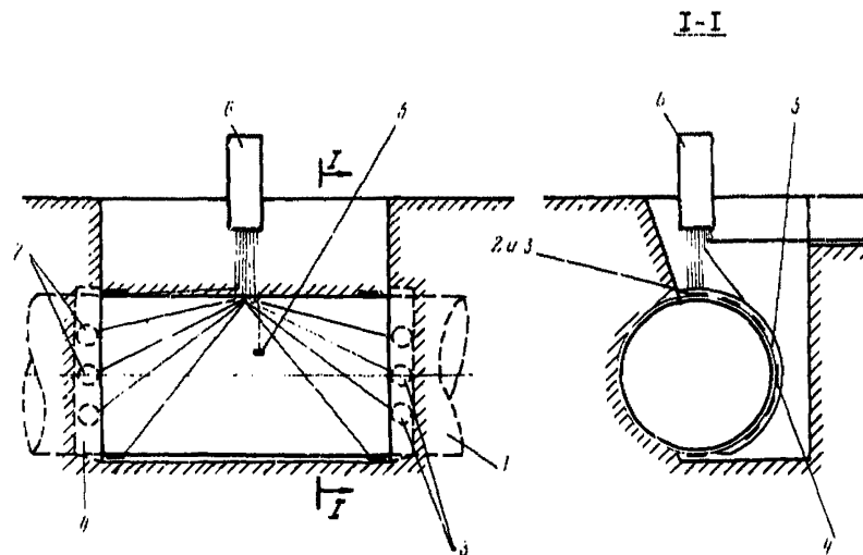
Рис. 5. Размещение оборудования в основном одностороннем нутре на трубопроводе большого диаметра:
