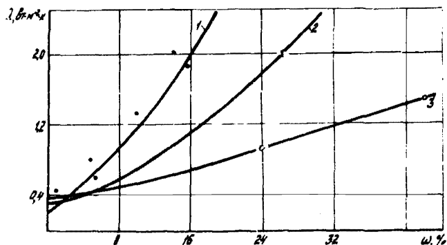
Рис. 4. Зависимость величины коэффициента теплопроводности грунта \lambda от влажности \omega :
