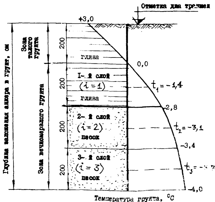
Рис.3. График распределения температур в грунте под трубопроводом
