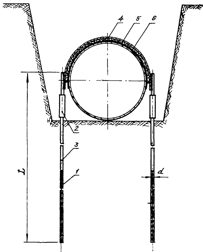
Рис.1. Стержневое анкерное устройство
