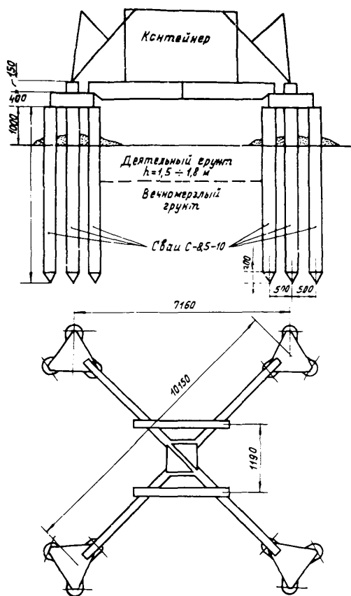
Рис.3. Фондамент башии РРЛ
