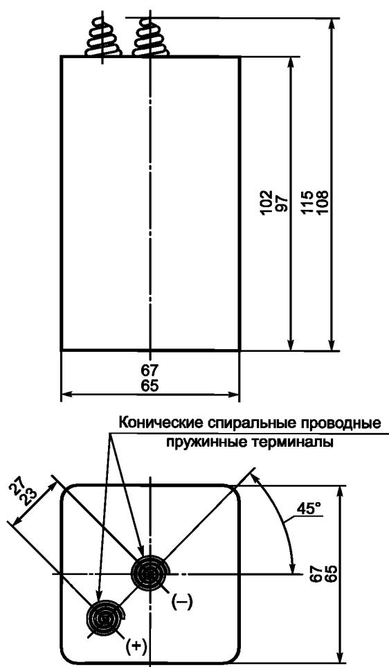
Рисунок 15 — Размеры батарей 4R25X, 4LR25X
