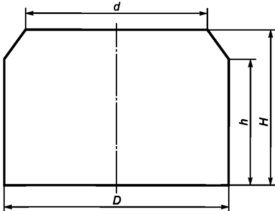
Рисунок 5 — Измерительный калибр для батарей категории 4
