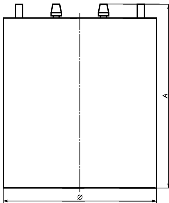
Рисунок 8 — Размеры батареи 5AR40
