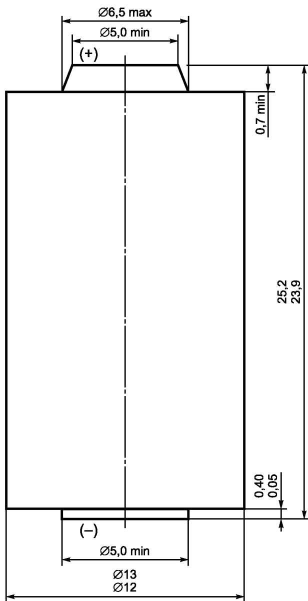
Рисунок 7 — Размеры батарей 4LR44, 2CR13252, 4SR44
