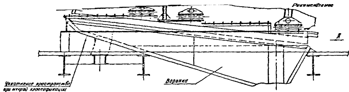
Вид А при мокрой классификации
