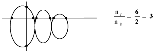
Рисунок 4.4. Определение кратности частот по фигурам Лиссажу.
