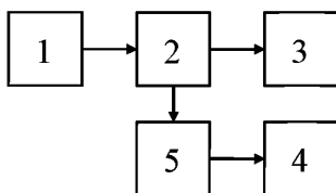
Рисунок 4.1. Структурная схема измерения частоты радиопередатчиков с применением электронно-счетных частотомеров.
