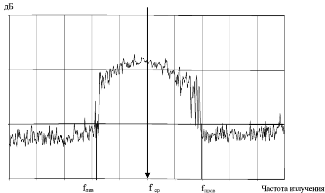
Рисунок 5 – Иллюстрация метода определения f_{ср}
