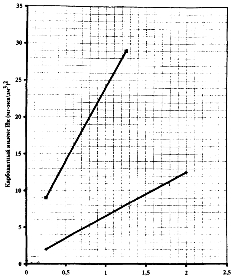
Рис. 3 Область применения ОЭДФК, АФОН 200-60А и их аналогов, проверенных и сертифицированных в РАО «ЕЭС России», для систем теплоснабжения при температуре 101-135°С и нагреве в водогрейных водотрубных котлах
