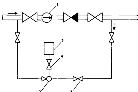
Рис. 19 Принципиальная схема установки дозирования с эжектором.
