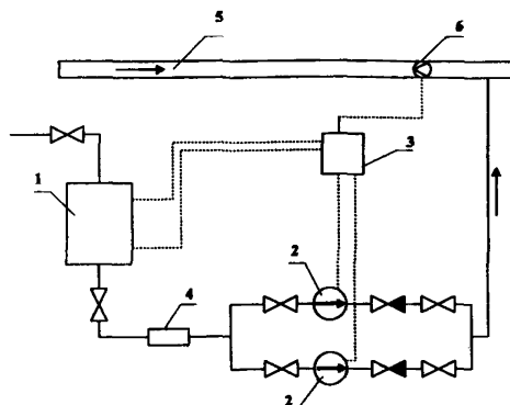
1 – расходный бак реагента; 2 – насос-дозатор; 3 – блок управления; 4 – фильтр; 5 – стационарный трубопровод; 6 – расходомер.
