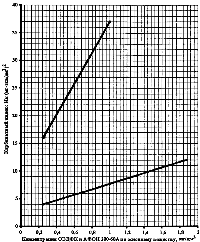
Рис.2 Область применения ОЗДФК, АФОН 200-60А и их аналогов, проверенных и сертифицированных в РАО «ЕЭС России», для систем теплоснабжения и ГВС при температуре не более 100°С и нагреве в водогрейных водотрубных котлах
