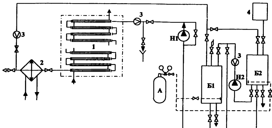
1 – секционированный водоводяной или пароводяной теплообменник типа "труба в трубе"; 2 – холодильник; 3 – расходомер; 4 – бак рабочего раствора антинакипина; Б1 – расходный бак; Б2 – бак подпиточной воды; Н1 – циркуляционный насос; Н2 – подпиточный насос; А – баллон с аргоном.
