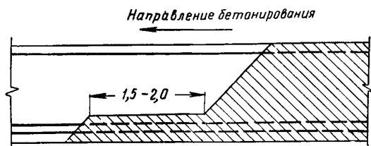
Рис. 7. Схема бетонирования балочных конструкций
