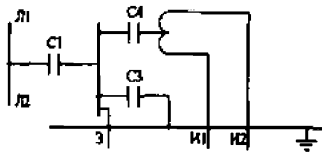
в) серия ТФЗМ (ТФН);
