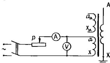
Рисунок Е.1 Схема измерения тока холостого хода трансформаторов напряжения.
