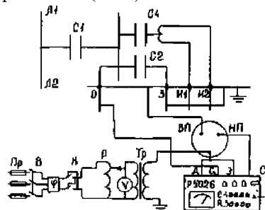
б) изоляции последних слоев по перевернутой схеме
