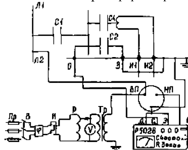
а) основной изоляции по нормальной схеме
