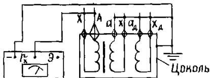
Рисунок Д.1 Схема измерения сопротивления изоляции первичных обмоток трансформаторов напряжения.
