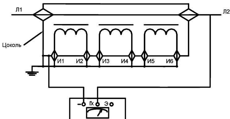
Рисунок В.1 – Схема измерения сопротивления изоляции первичных обмоток ТТ.
