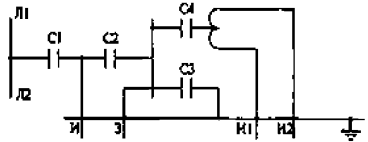
б) типа ТФКН-330
