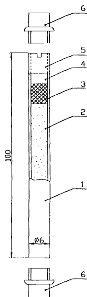
Рис.1 Колонка накопительная
