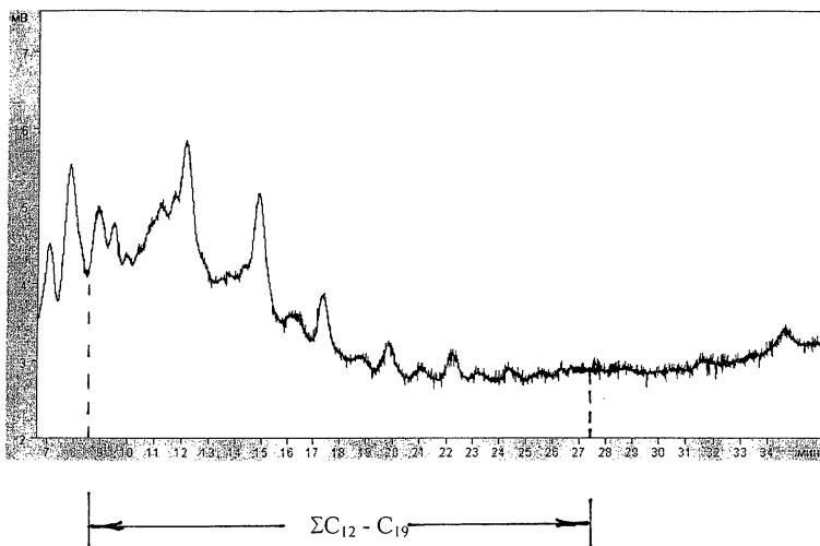
Рис.3. Хроматограмма экстракта пробы углеводородов C_{12}-C_{19} , отобранных из мазутохранилища при 50^{\circ}C ( \Sigma C_{12-C_{19}} = 26,7 \text{ мг/м}^3 )
