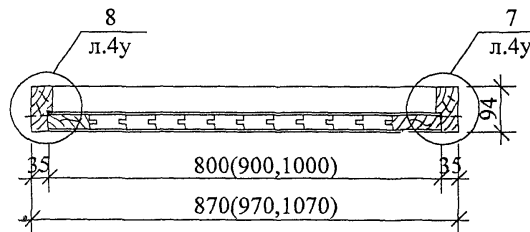
A - A (ОАО "Заречье", ОАО "ДОК №5")
