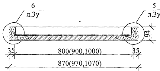
A - A (ОАО "Заречье", ОАО "ДОК №5")
