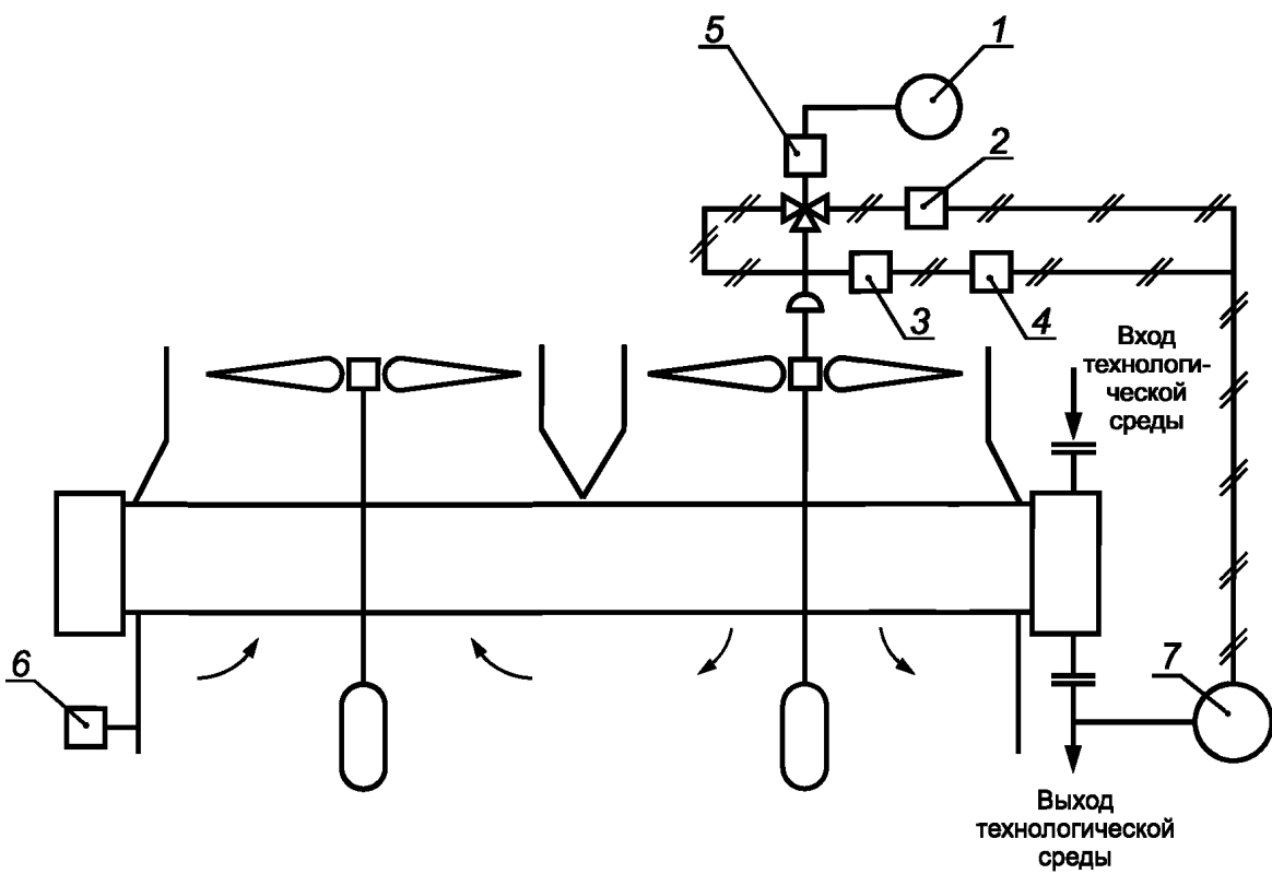
1 — выключатель по температуре окружающего воздуха; 2 — реле верхнего предела; 3 — реверсирующее реле; 4 — реле нижнего предела; 5 — трехходовой электромагнитный переключатель; 6 — ветровой экран; 7 — контроллер с индикацией температуры
