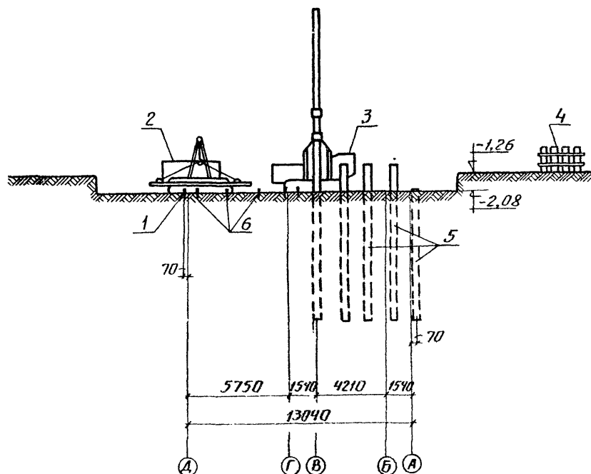
Рис.7. Поперечный разрез свайного поля: 1-места положения свай главных осей; 2-трубо- укладчик ТД-Т-75; 3-сваебойный агрегат С-878М; 4-штабеля свай; 5-забитые сваи; 6-места поло- жения свай промежуточных осей
