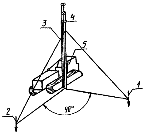
Рис.12. Схема выверки вертикальности сваи отвесами: 1-отвес закопёрщика; 2-отвес копровщика; 3-свая; 4-оголовок; 5-сваебойный агрегат С-878М
