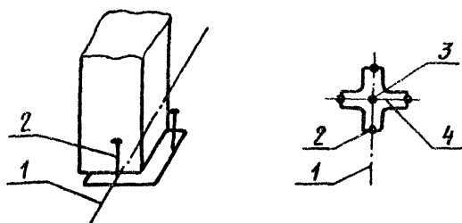
Рис.10. Схема установки свай на точку: 1-ось свайного ряда; 2-разметочный штирь; 3-установочный штирь, 4-шаблон
