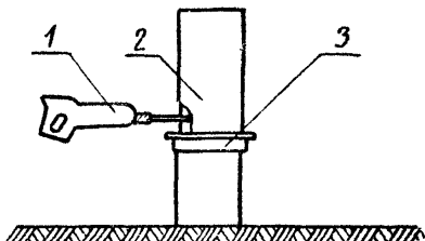
Рис.17. Схема срубке голов свай: 1-пневматический молоток; 2-свая; 3-обжимной хомут
