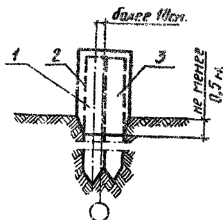
Рис.19. Исправление дефектов при отклонении свай более 10 см: 1-забитая свая, с отклонением; 2-моноклитическая насадка; 3-свая-дублер
