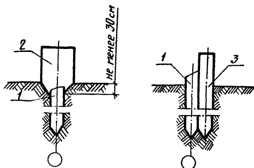
Рис.20. Исправление дефектов при поломке свай: 1-забитая сломанная свая; 2-насадка из сборной оболочки \varnothing 80 см; 3-свая-дуплер
