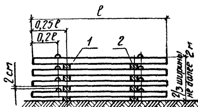
Рис.5. Схема укладки свай в штабель: 1-сваи; 2-деревянные прокладки из бруса 100х100 мм
