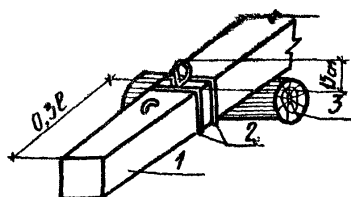
Рис.9. Строповка сваи для подъема под наголовник: 1-свая; 2-кольцевой строп; 3-подкладка
