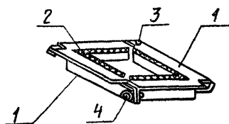
Рис.16. Обжимной хомут: 1-уголок 75х75; 2-резиновая прокладка; 3-шарнир; 4-болт \varnothing 20 мм
