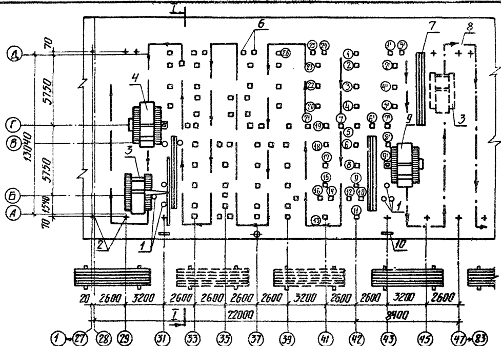
Рис. 6. Схема забивки свай: 1-места расположения свай; 2-места расположения свай на главных осях; 3-трубоукладчик ТД-Т-75; 4-сваебойный агрегат С-878М № 1; 5-направление движения агрегата № 1; 6-забитые сваи; 7-разложенные сваи; 8-направление движения агрегата № 2; 9-сваебойный агрегат С-878М № 2; 10-переносные визирки; 1 2 3 - последовательность забивки свай агрегатом № 1; ① ② ③ - последовательность забивки свай агрегатом № 2
