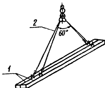
Рис.8. Схема строповки свай при раскладке: 1—свая; 2—четырёхветвевой строп грузоподъемностью 5 т
