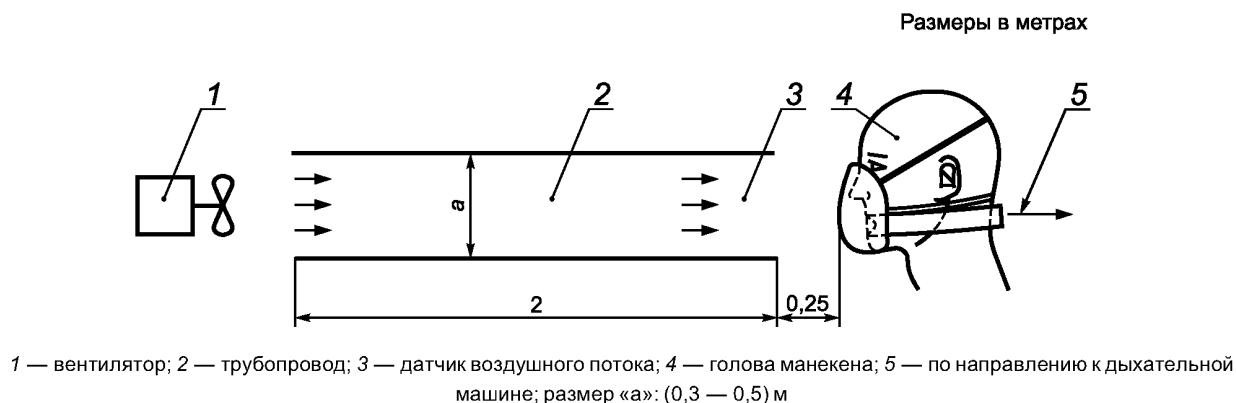
Рисунок 7 — Схема проведения испытания по определению содержания диоксида углерода
