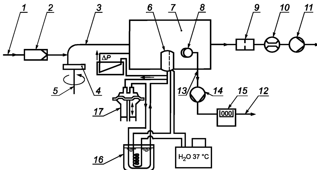
1 — сжатый воздух; 2 — воздушный фильтр; 3 — инжектор; 4 — доломитовый порошок; 5 — пылеподачик; 6 — испытуемый образец; 7 — испытательная камера; 8 — пробоотборник; 9 — фильтр; 10 — расходомер; 11 — насос; 12 — отвод воздуха; 13 — линия пробоотбора; 14 — насос; 15 — счетчик; 16 — сатуратор; 17 — дыхательная машина
