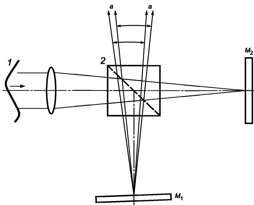
1 — асферический волновой фронт; 2 — светоделитель; M_1 — первое зеркало; M_2 — второе зеркало; а — излучение, направленное к приемнику
