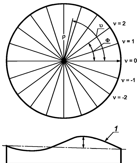
Рисунок 22 — Одна из трех поверхностей A, B или C (вид сверху и сбоку)
