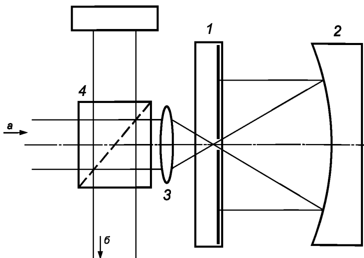
1 — плоское зеркало; 2 — параболюид; 3 — формирующая оптическая система; 4 — поляризационный светоделитель; а — излучение лазера; б — излучение, направленное к приемнику
