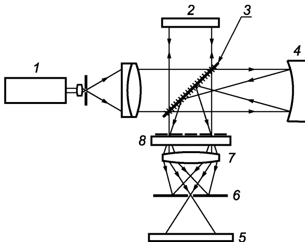
1 — лазер; 2 — опорное зеркало; 3 — светоделиватель; 4 — параболическое зеркало; 5 — плоскость интерференции; 6 — пространственный фильтр; 7 — формирователь изображения; 8 — осесимметричная голограмма
