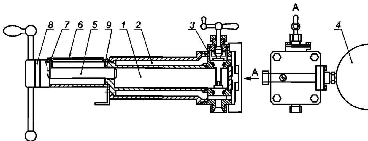
1 — пробоотборная камера; 2 — термостатирующая рубашка; 3 — клапанный узел; 4 — манометрический узел; 5 — плунжер; 6 — линейная шкала; 7 — визир; 8 — лимб; 9 — корпус
