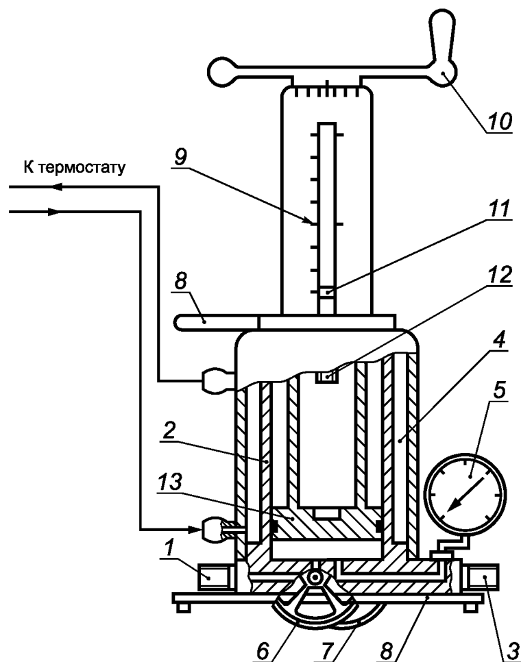
1 — входной штуцер; 2 — цилиндр; 3 — выходной штуцер; 4 — термостатирующая рубашка; 5 — манометр; 6 — входной вентиль; 7 — выходной вентиль; 8 — установочные опоры; 9 — линейная шкала; 10 — штурвал; 11 — визир; 12 — ходовой винт; 13 — шток с поршнем
