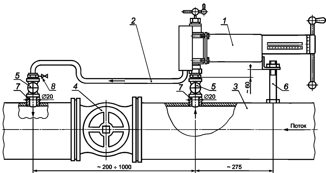
1 — прибор УОСГ-100 СКП; 2 — соединительный шланг; 3 — трубопровод; 4 — задвижка (местное гидравлическое сопротивление); 5 — вентиль D_y 20 (R^{3/4}) ; 6 — болт М 16; 7 — входной и выходной штуцера; 8 — кран
