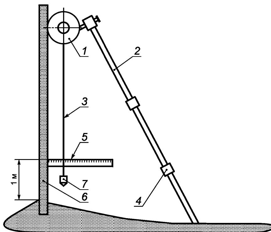
1 — каретка; 2 — штанга составная (труба 1\frac{1}{2} — 3\frac{3}{4} )*, l = 5 - 6 м; 3 — капроновая нить \varnothing 0,7 - 0,8 мм; 4 — муфта соединительная; 5 — линейка по ГОСТ 427; 6 — внутренняя стенка резервуара; 7 — груз
