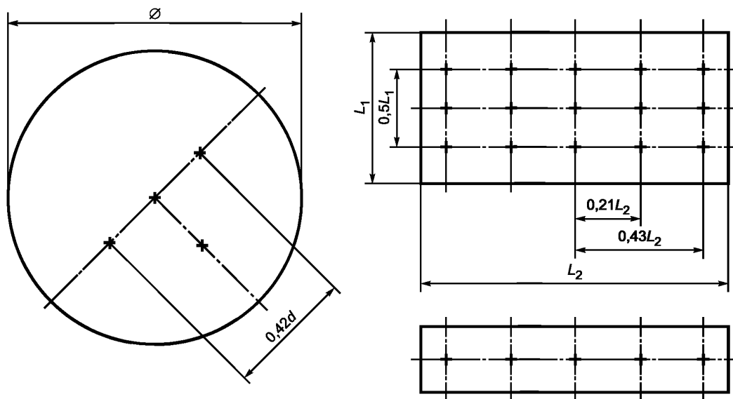
Рисунок 4 — Размещение датчиков для измерения температуры
