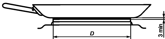
Рисунок 6 — Кастрюля
