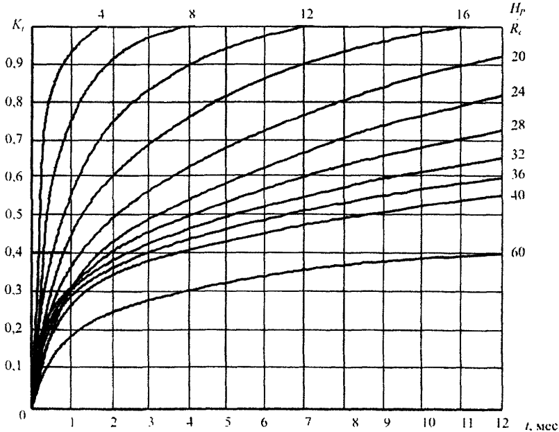
Рисунок Е.5 – Графики для определения коэффициента K_i при t менее одного года
