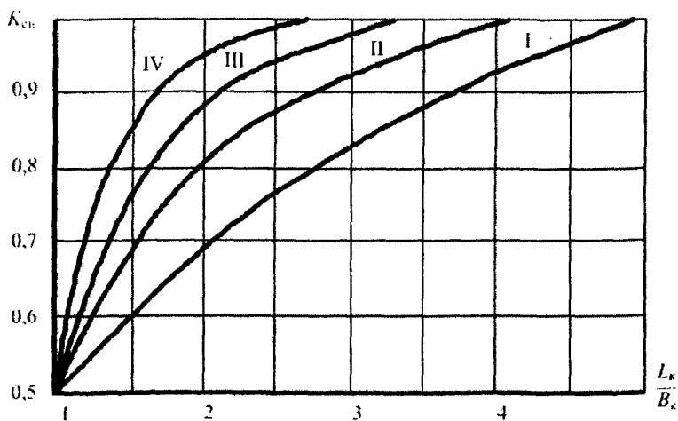
Рисунок Е.6 — Графики для определения коэффициента k_{сн}
