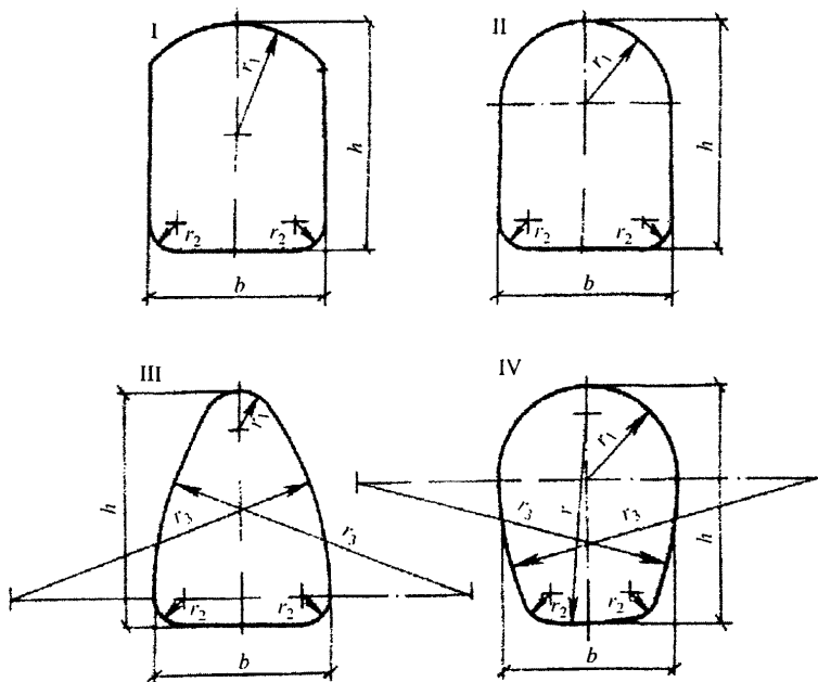
Рисунок 1 – Формы поперечных сечений безнапорных туннелей в свету
