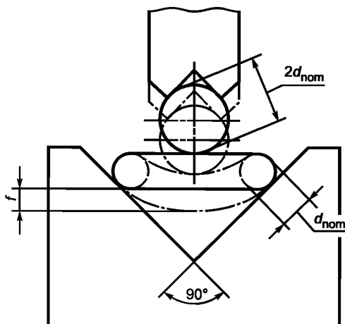
Рисунок 1 — Прогиб f
