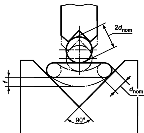
Рисунок 1 — Прогиб f
