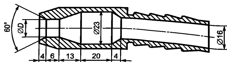
Рисунок А.5 — Ручное устройство для проверки защиты от дождевания и разбрызгивания воды
