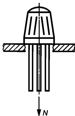
Рисунок 106 — Пример приложения усилия натяжения по оси зажима
