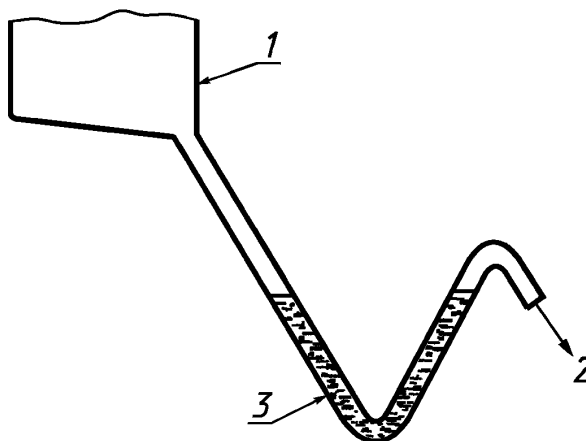
1 — распылитель; 2 — отходы; 3 — вода, образующая газовый замок
