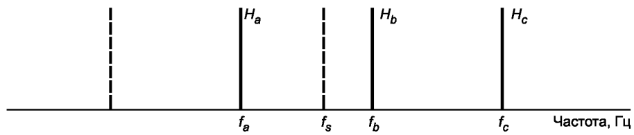
Рисунок G.1 — Примеры выбора частоты H_c
