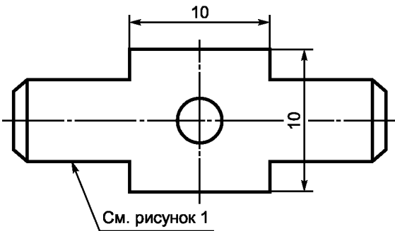
Рисунок 6 — Двухконцевой штекер
