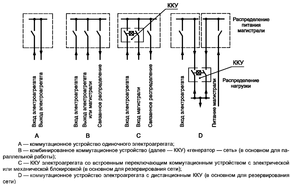
Рисунок 1 — Схемы коммутационных устройств электроагрегатов
