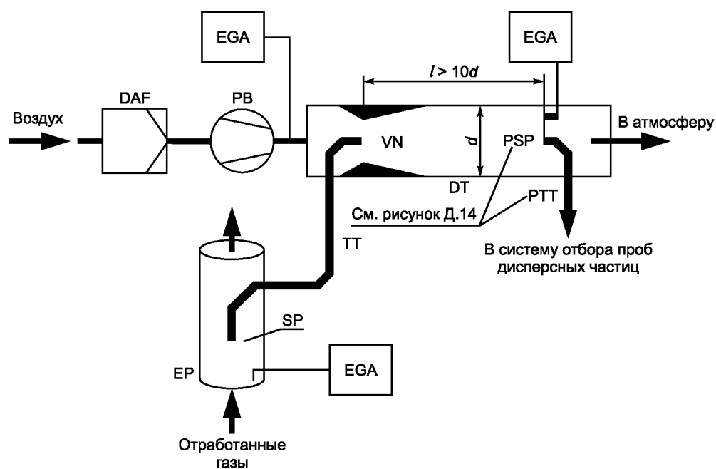
Рисунок Д.8 — Система с частичным разбавлением потока, частичным отбором проб, одинарной трубкой Вентури и измерением концентрации \text{CO}_2 или \text{NO}_x
