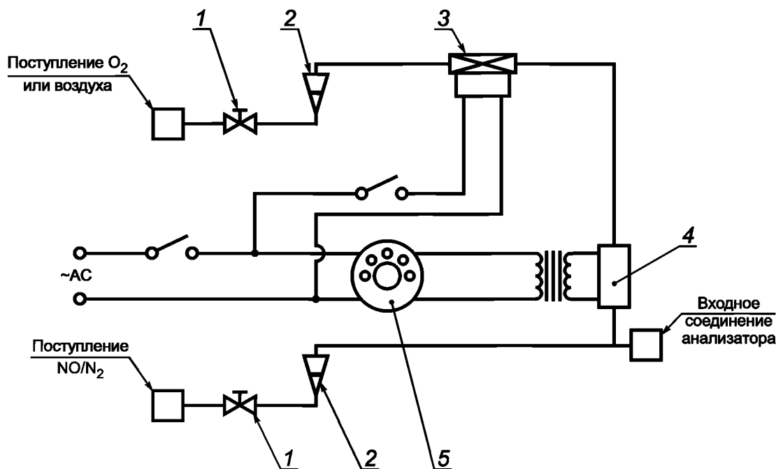
1 — клапан управления расходом; 2 — расходомер; 3 — электромагнитный клапан управления расходом; 4 — озоногенератор; 5 — вариатор
