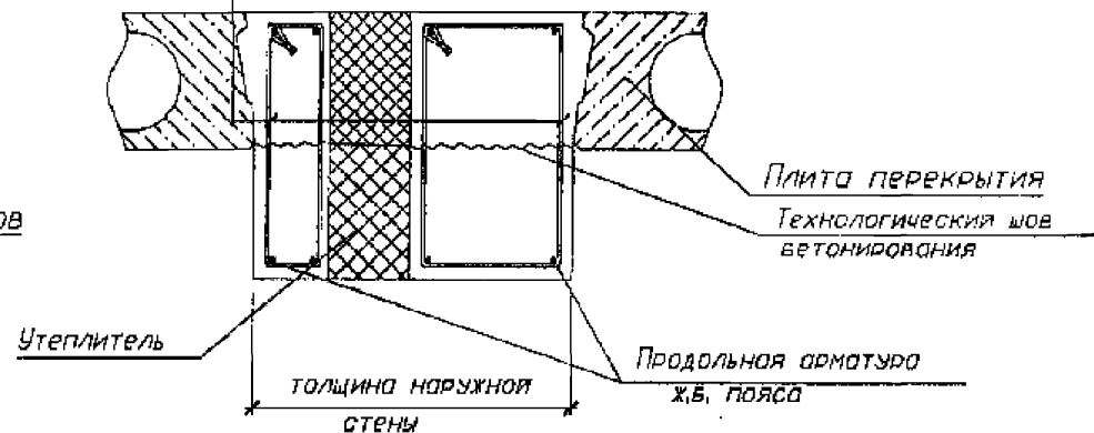
3-3 (по утеплителю)
