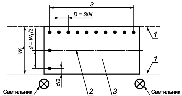
1 — край дороги; 2 — центральная линия дороги; 3 — контрольный участок
