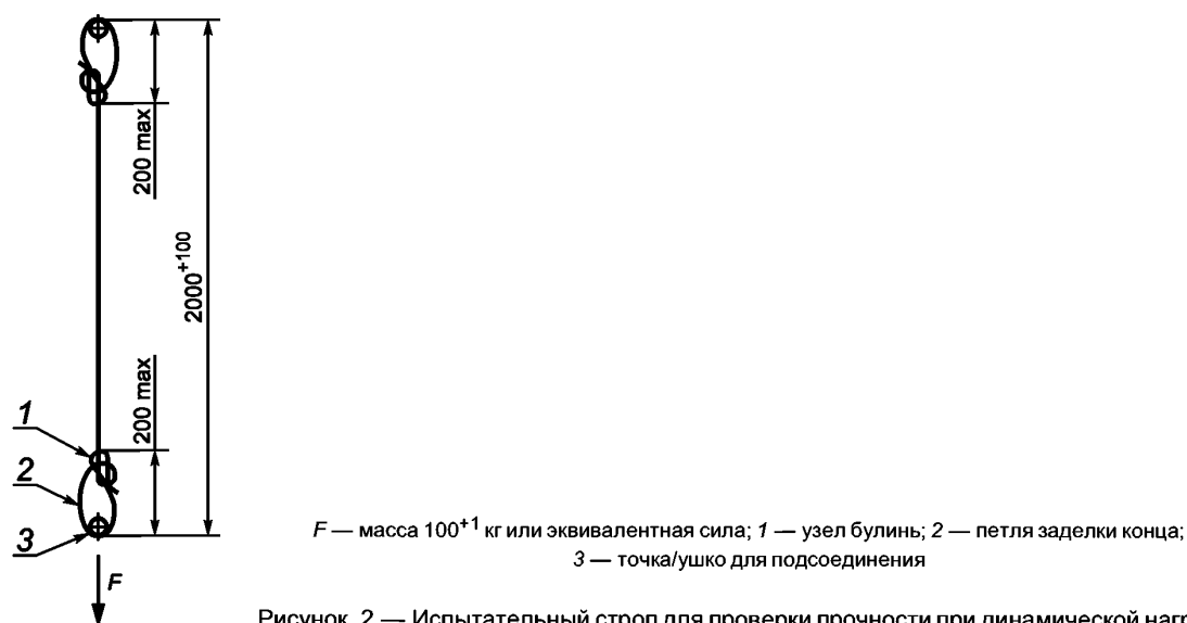
Рисунок 2 — Испытательный строп для проверки прочности при динамической нагрузке
