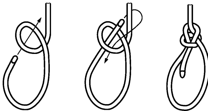
Рисунок 5 — Узел булинь
