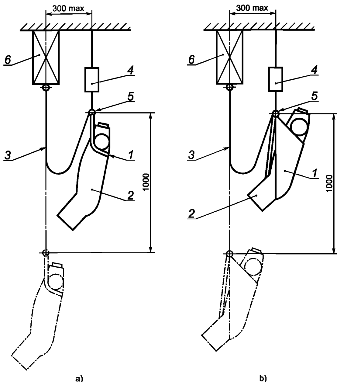
а) — класс А; б) — класс В; 1 — спасательная петля; 2 — манекен корпуса человека; 3 — испытательная стропа; 4 — устройство быстрого расцепления; 5 — элемент крепления; 6 — испытательное оборудование
