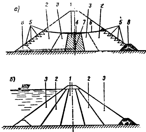
Рис. 1. Наименования отдельных частей и элементов земляной намывной плотины
