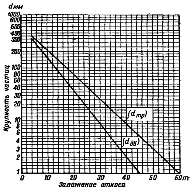
Рис. 4. График для определения крупности частиц пригрузки при нефронтальном действии волн ( \psi = 45^\circ ) высотой 1 м
