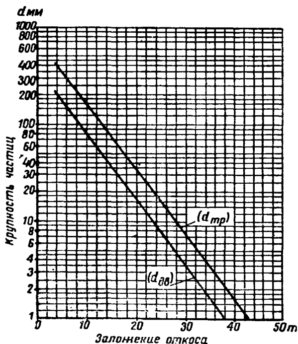
Рис. 3. График для определения крупности частиц пригрузки при фронтальном действии волн ( \psi = 90^\circ ) высотой 1 м
