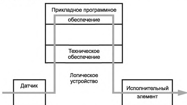
Рисунок С.1 — Логическое решающее устройство
