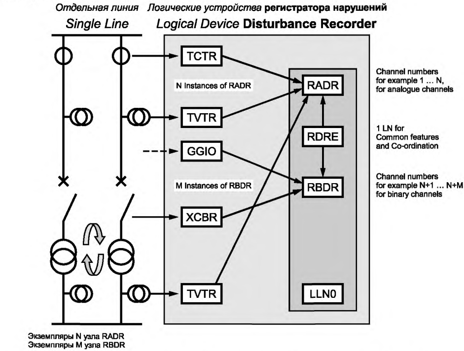
Номера каналов для примера 1 ... N — для каналов передачи аналоговых данных 1 логический узел для общих свойств и координирования Номера каналов для примера N+1 ... N+M — для каналов передачи двоичных данных
