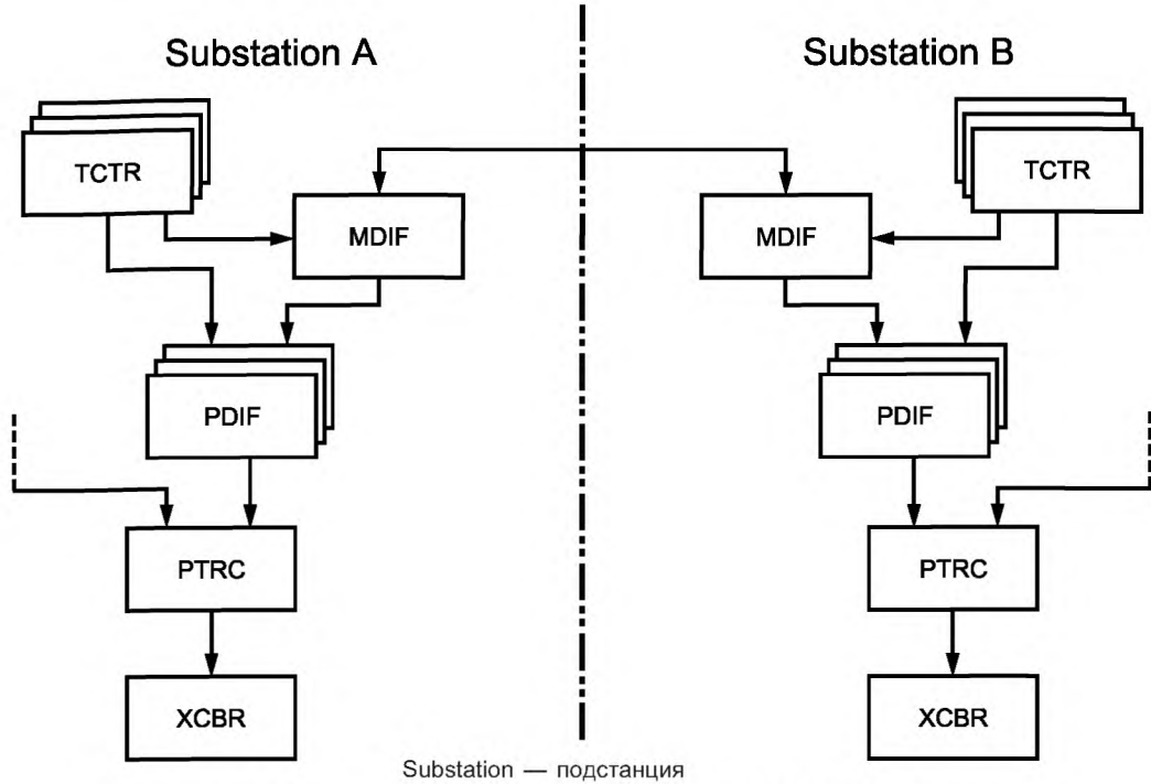
Рисунок В.3 — Использование логических узлов MDIF и PDIF
