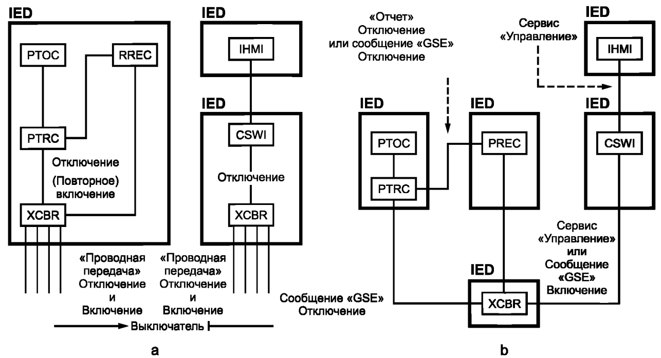
Рисунок B.7 — Использование логического узла RREC
