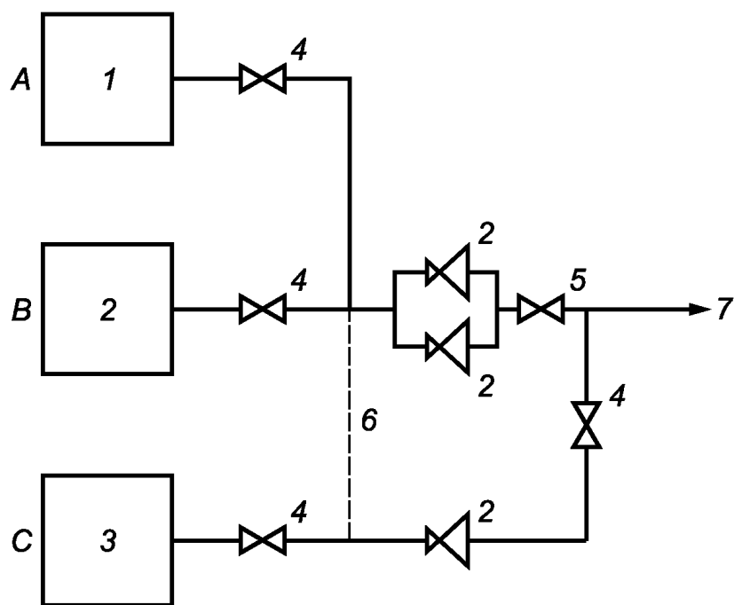
А — первичный источник подачи; В — вторичный источник подачи; С — резервный источник подачи; 1 — блок(и) концентратора кислорода; 2 — регулятор давления трубопровода; 3 — две группы баллонов высокого давления; 4 — запорный вентиль источника подачи; 5 — запорный вентиль системы подачи; 6 — необязательное соединение; 7 — к отводящей трубопроводной системе
