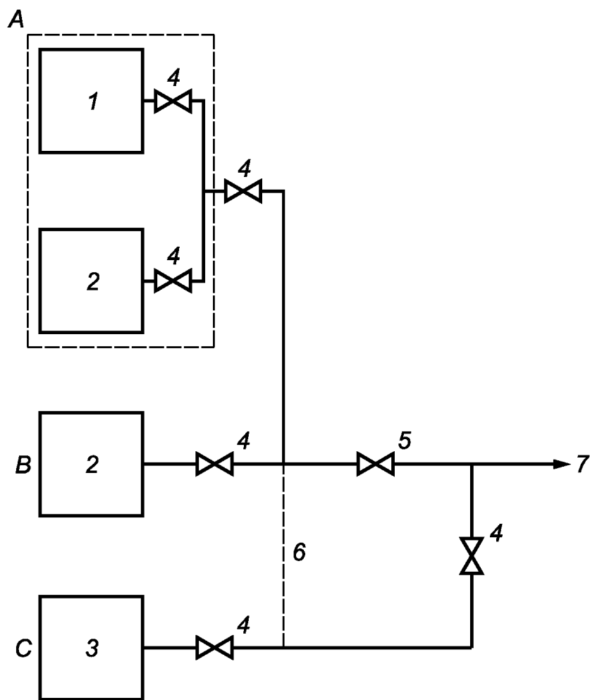
А — первичный источник подачи; В — вторичный источник подачи; С — резервный источник подачи; 1 — блок(и) концентратора кислорода; 2 — баллоны высокого давления, содержащие кислород или воздух, обогащенный кислородом, или криогенный сосуд(ы) для жидкости; 3 — две группы баллонов высокого давления; 4 — запорный вентиль источника подачи; 5 — запорный вентиль системы подачи; 6 — необязательное соединение; 7 — к отводящей трубопроводной системе
