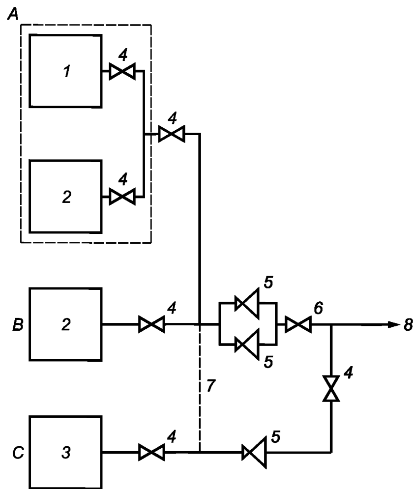
A — первичный источник подачи; B — вторичный источник подачи; C — резервный источник подачи; 1 — блок концентратора кислорода; 2 — баллоны высокого давления, содержащие кислород или воздух, обогащенный кислородом, или криогенный сосуд для жидкого кислорода; 3 — две группы баллонов высокого давления; 4 — запорно-выпускной вентиль источника подачи; 5 — регулятор давления трубопровода; 6 — запорный вентиль системы подачи; 7 — необязательное соединение; 8 — к отводящей трубопроводной системе Рисунок А.3 — Системы подачи с концентратором кислорода с одним блоком концентратора кислорода и дополнительными баллонами высокого давления или криогенным сосудом(и) для жидкости первичного источника, баллонами высокого давления или криогенным сосудом для жидкости вторичного источника и баллонами высокого давления резервной системы для одноступенчатой распределительной системы
