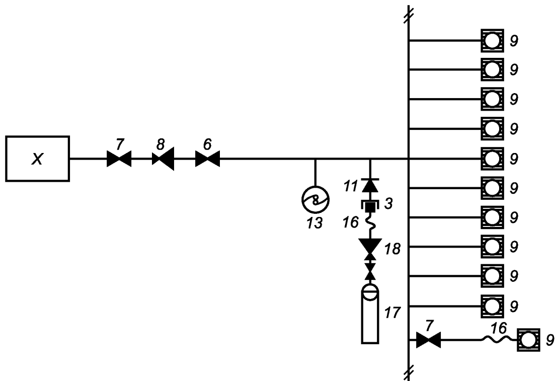
Рисунок A.29 — Местная распределительная система для двухступенчатой трубопроводной распределительной системы с двумя параллельными регуляторами давления
