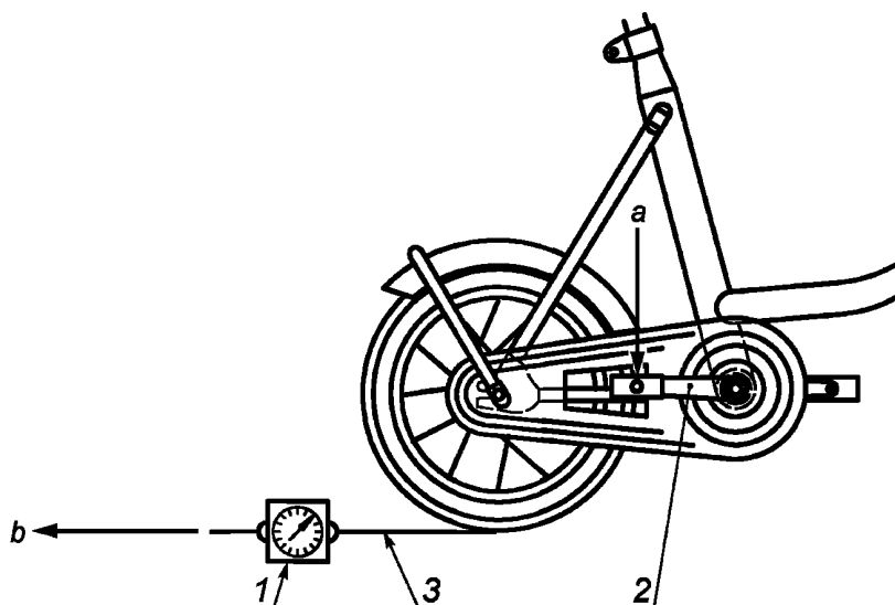
1 — механизм измерения силы; 2 — правый шатун; 3 — соответствующая лента, оборачиваемая вокруг окружности колеса; а — направление прикладываемой силы на педаль; b — прикладываемая сила на колесо (сила торможения)
