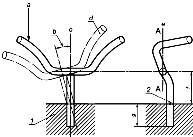
1 — зажимное приспособление; 2 — ограничительная метка; a — прикладываемый момент кручения; b — остаточная деформация; c — ось стержня; d — отклонение формы; e — прикладываемый момент кручения в сечении А—А; f — длина свободного стержня; g — минимальная глубина ввода
