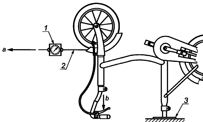
1 — механизм измерения силы; 2 — соответствующая лента, оборачиваемая вокруг окружности колеса; 3 — зажимное приспособление; а — прикладываемая сила на колесо (сила торможения); b — прикладываемая сила на рукоятку
