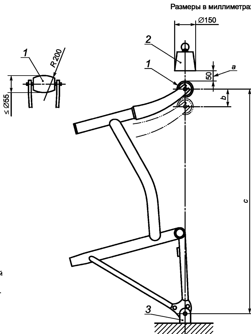
Рисунок 14 — Испытание на удар (падающая масса)
