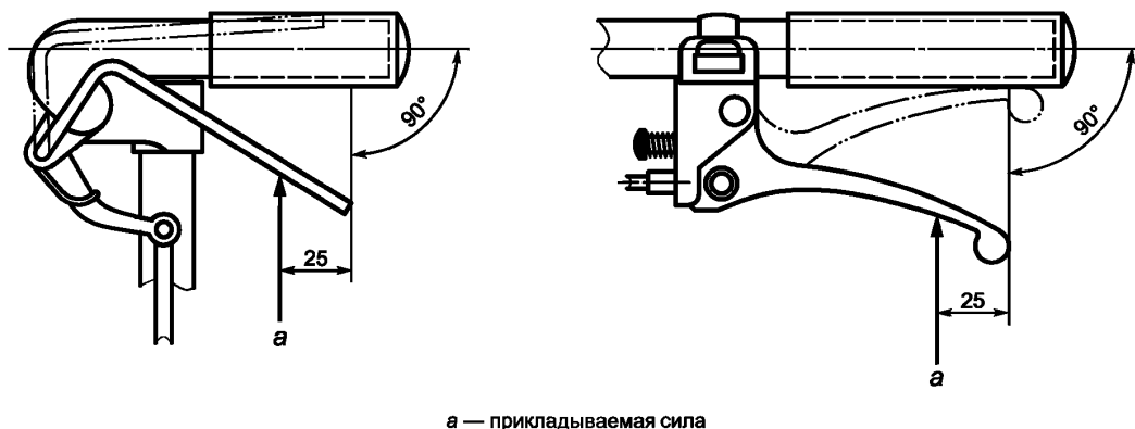
Рисунок 7 — Прикладываемая сила на рукоятках ручного тормоза
