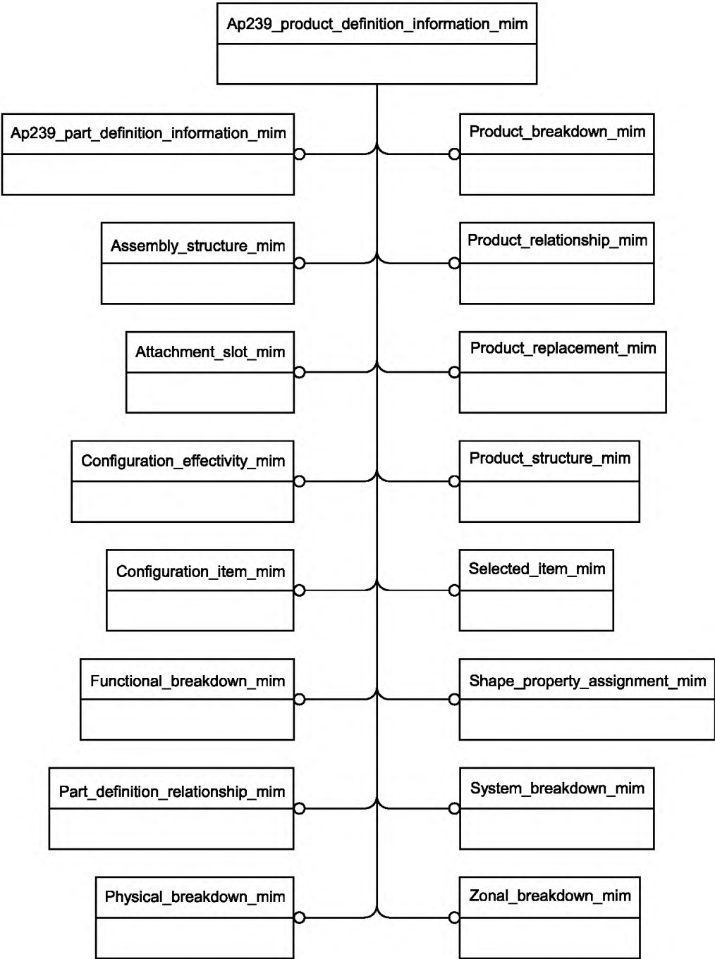
Рисунок D.1 — Представление ИММ на уровне схем в формате EXPRESS-G (диаграмма 1 из 1)
