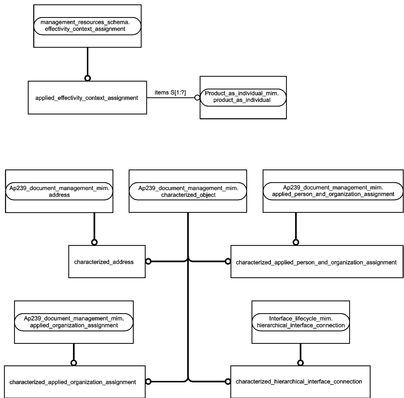
Рисунок D.2 — Представление IMM на уровне объектов в формате EXPRESS-G (диаграмма 1 из 2)
