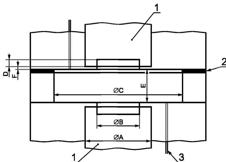
Рисунок С.2 — Эскиз камеры большого объема
