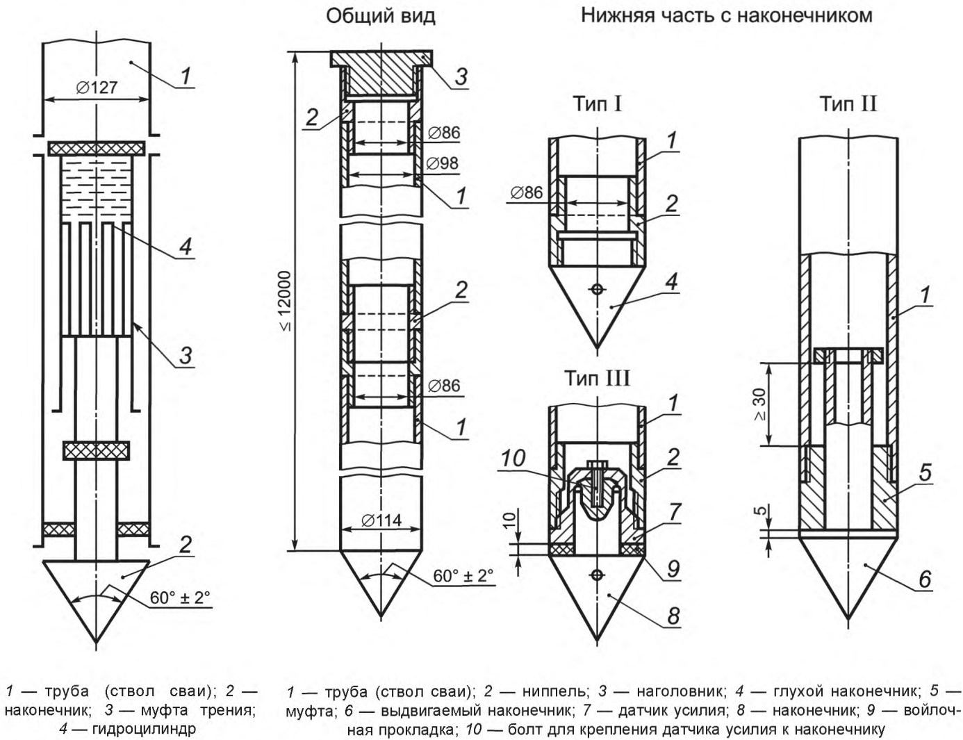
Рисунок В.1 — Схема конструкции сваи-зонда
