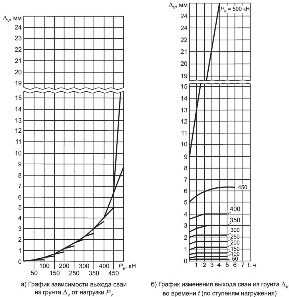
Рисунок Л.1 — Графики результатов испытаний грунтов выдергивающей нагрузкой натурной сваей
