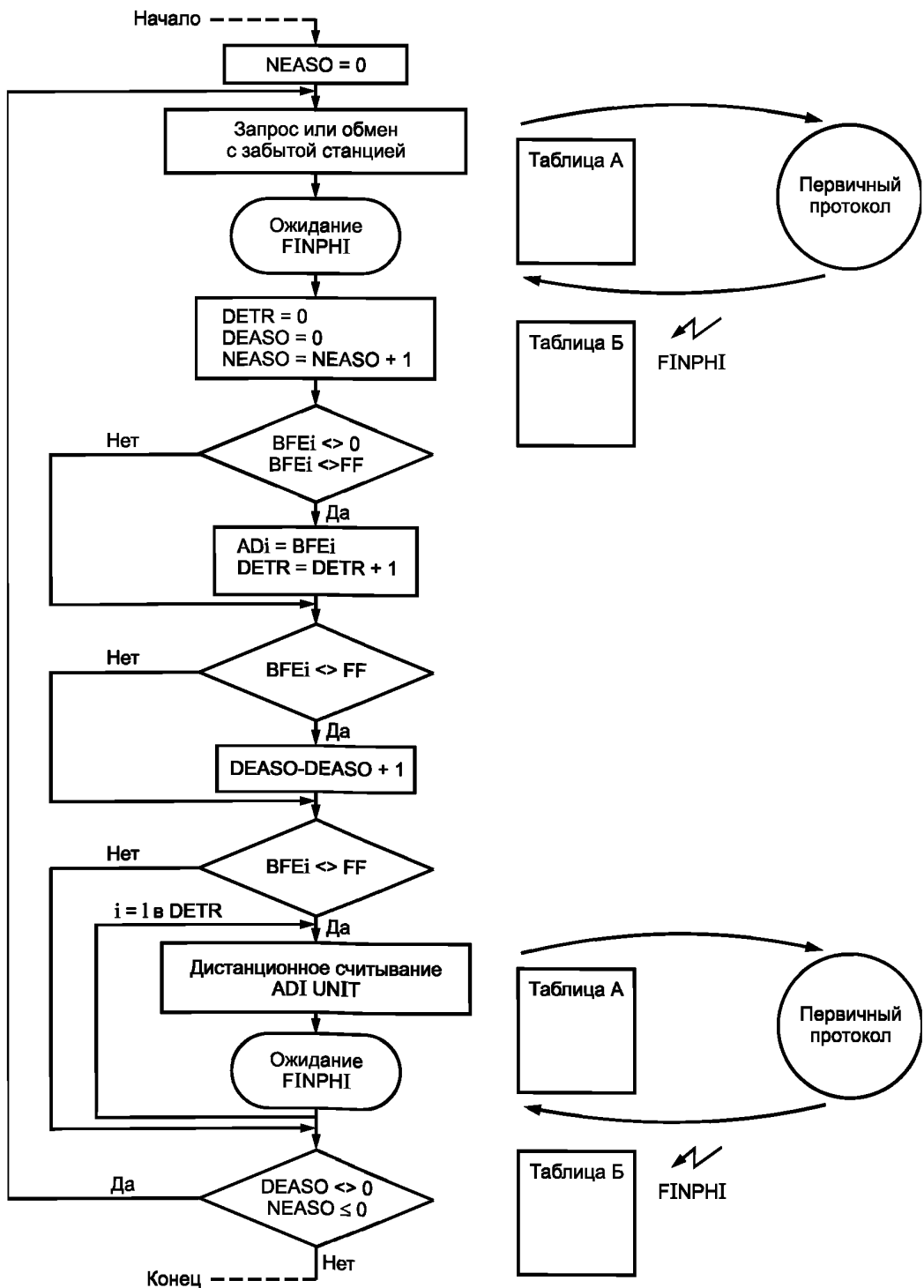
Блок-схема запроса забытой станции
