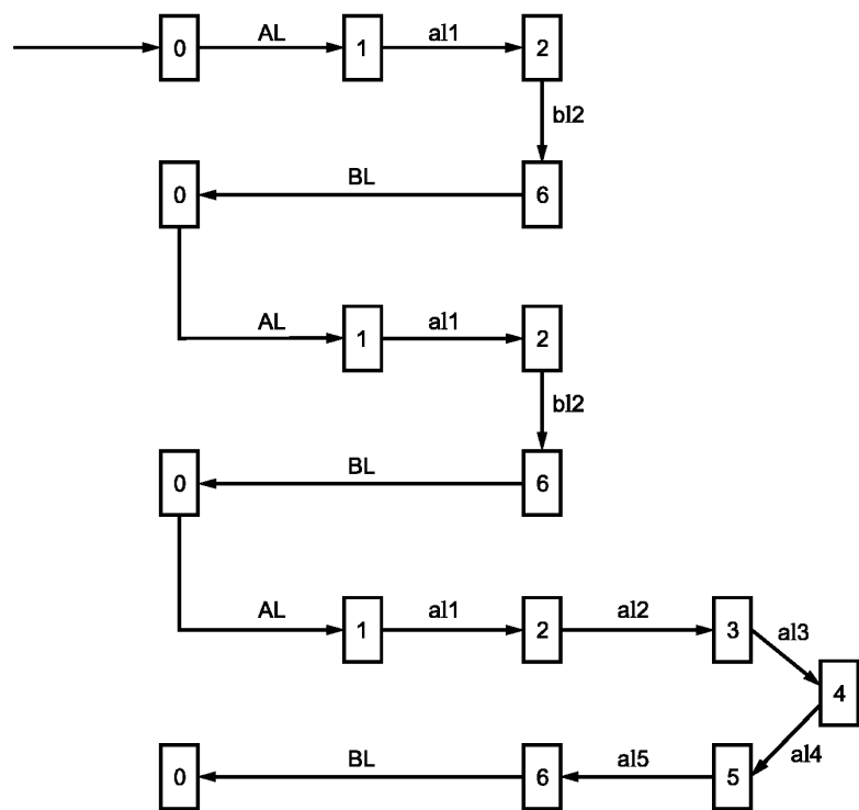
Пример перезапусков после ошибки и на СЕАНСОВОМ уровне (ERSES = 1), за которыми следует правильное дистанционное считывание с третьей попытки.
