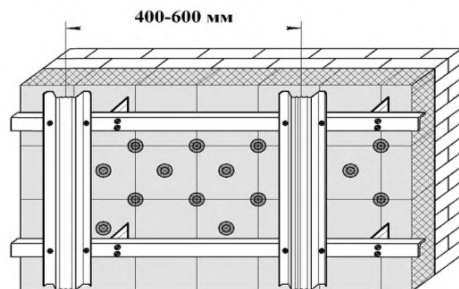
Рисунок 8 – Крепление направляющих профилей ПОП4
