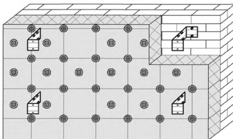
Рисунок 4 – Крепление утеплителя
