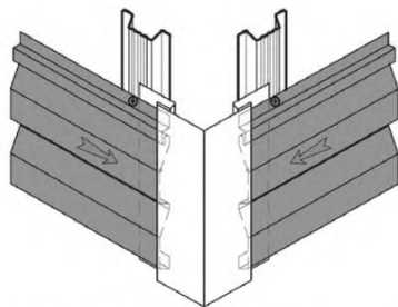
Рисунок 12 – Обрамление наружного угла. Накщельник угловой наружный ПОН4-1
