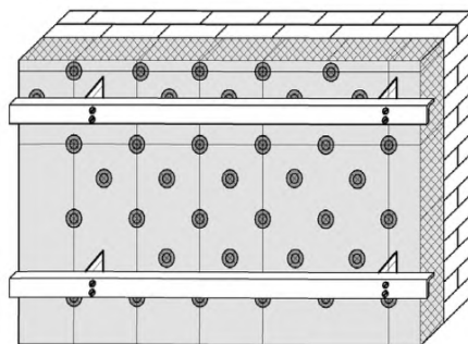
Рисунок 7 – Крепление горизонтальных профилей
