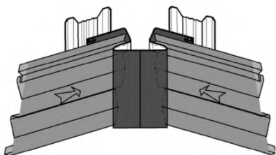
Рисунок 11 – Обрамление внутреннего угла. Накщельник угловой внутренний ПОНЗ-1
