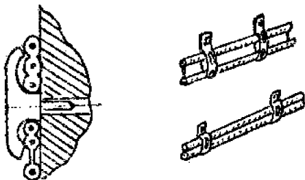
Рис.18. Крепление проводов
