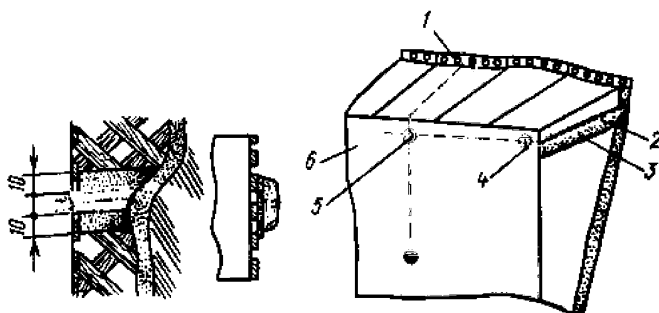
Рис.4. Скрытые электропроводки под горючими основаниями и в пустотах строительных конструкций:
