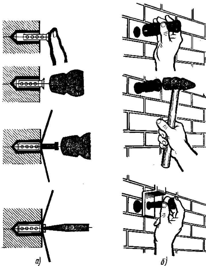
Рис.13. Последовательность операций установки и закрепления распорных дюбелей:
